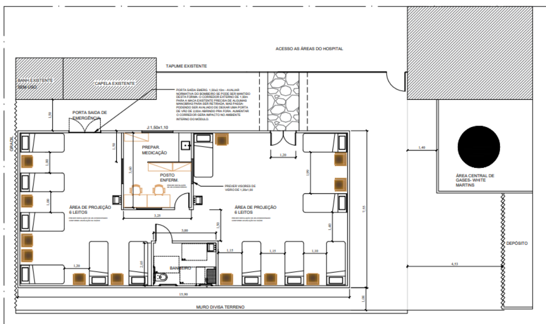
Imagem 01: Estudo Preliminar- Planta de layout Módulo Enfermaria
